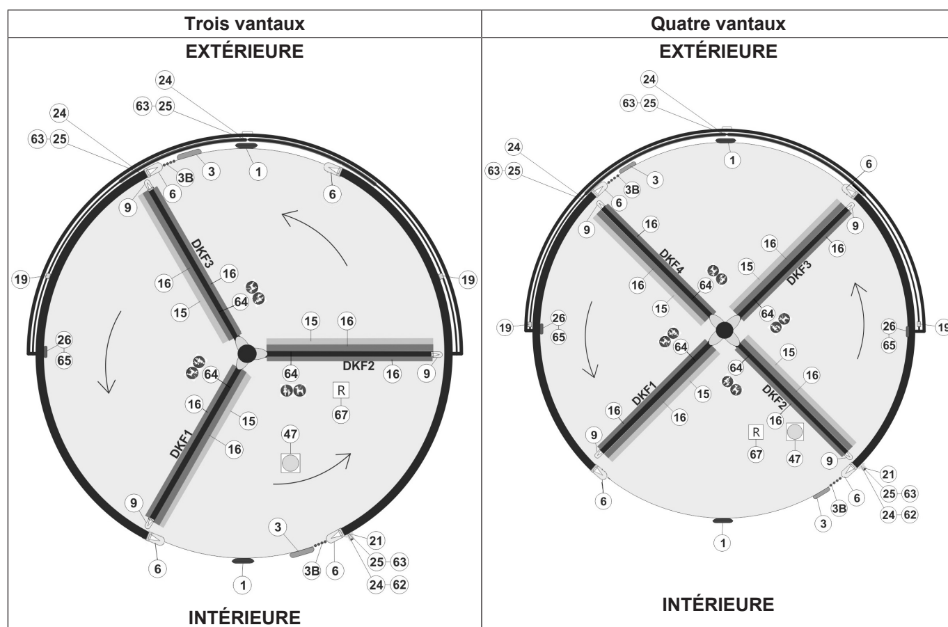
Positions des vantaux du tourniquet dans la position verrouillée:
